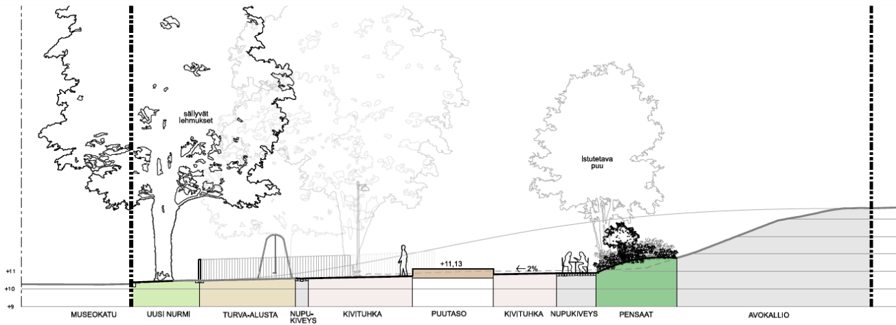
LEIKKAUS B-B' 1:200
