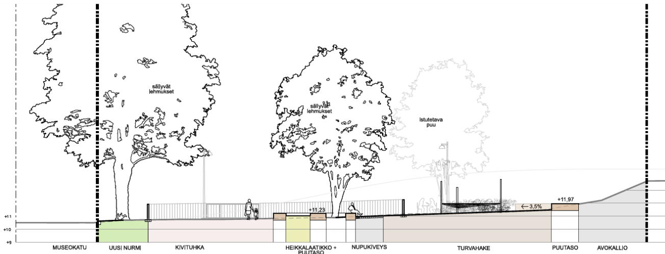
LEIKKAUS A-A' 1:200
