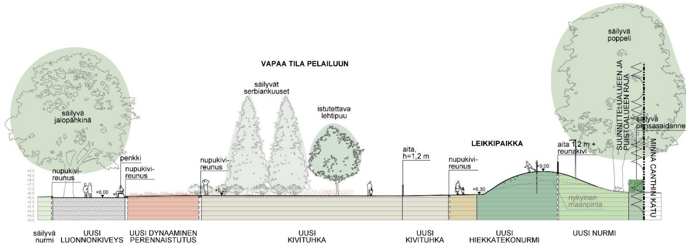
POIKKILEIKKAUS A-A'
