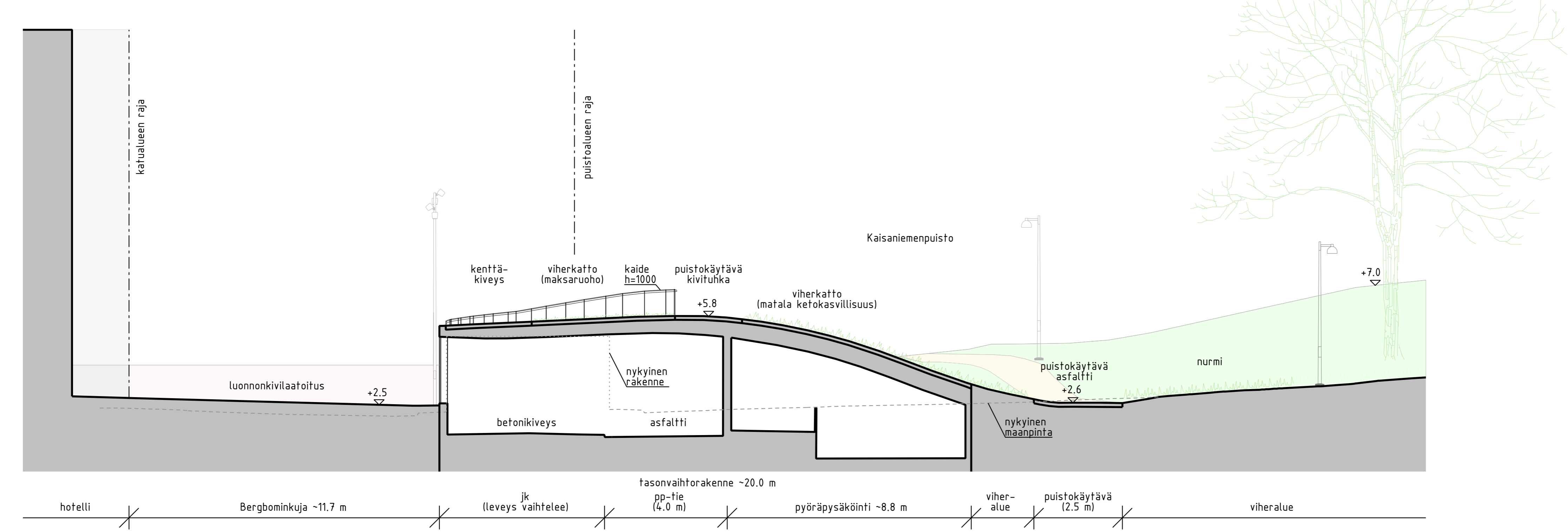
LEIKKAUS A-A 1:100
