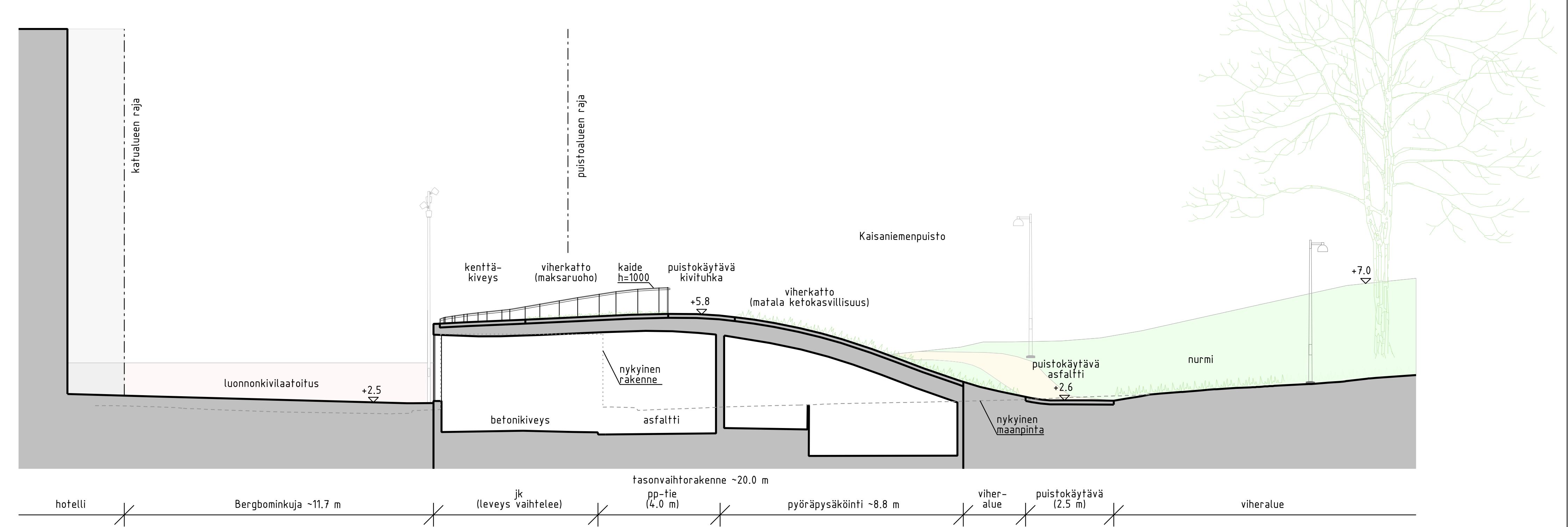
LEIKKAUS A-A 1:100
